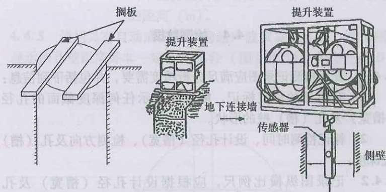
图4.3.2 超声波仪器架设示意图
